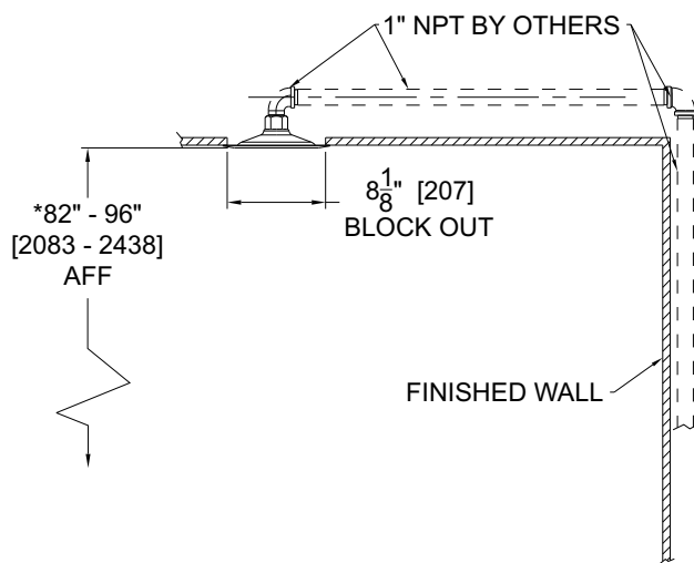
S3200-RA
