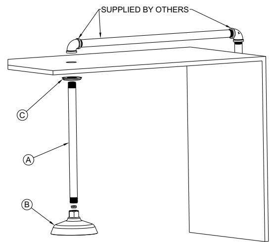
S2100-PE21-RA
